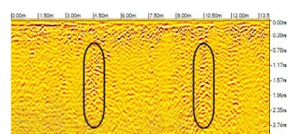
Мал. 18. Профіль 5. Аваламі паказана прыкладнае размяшчэнне лініі падмурка
