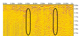
Мал. 16. Профіль 3. Аваламі паказана прыкладнае размяшчэнне лініі падмурка
