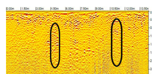
Мал. 17. Профіль 4. Аваламі паказана прыкладнае размяшчэнне лініі падмурка
